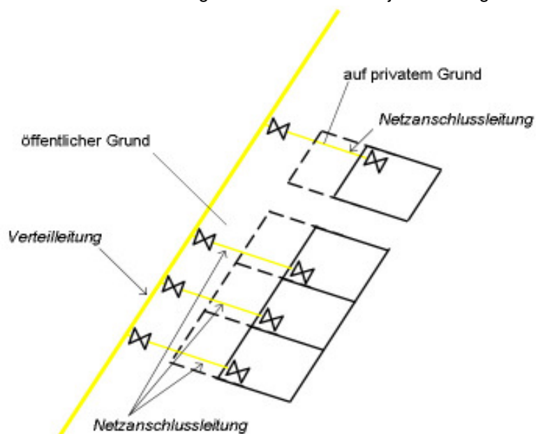
Schema Netzanschluss
